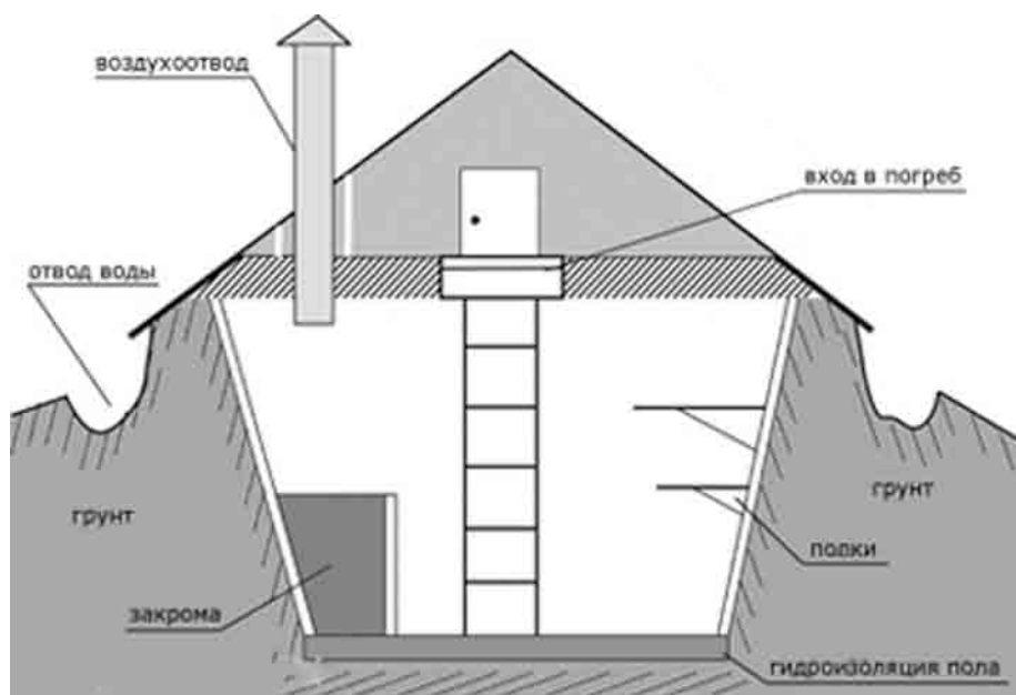
Схема постройки полуглубленного погреба
